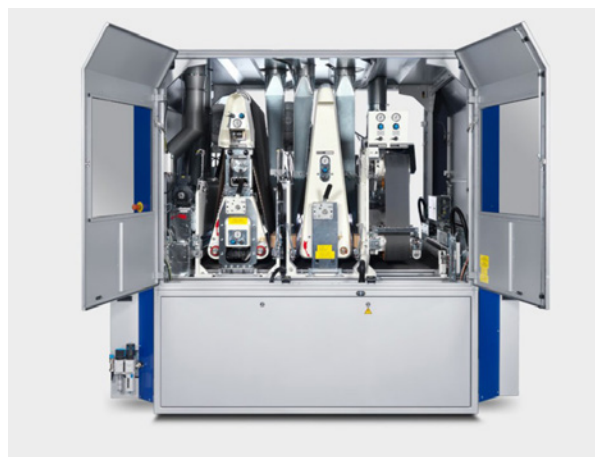
□ CSD sustav sa magnetom pritiskom gredom
